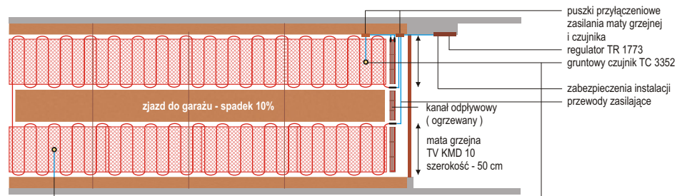
ogrzewanie zjazdu do garażu
